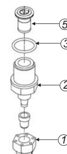
SUCTION 59-839-I
